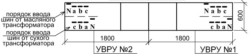
План расположения
